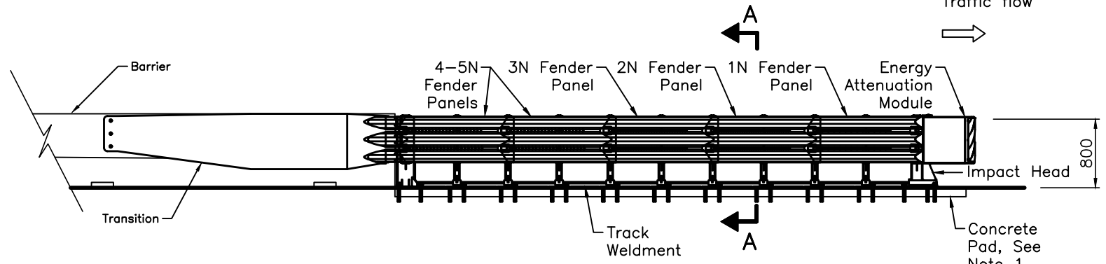
ELEVATION
