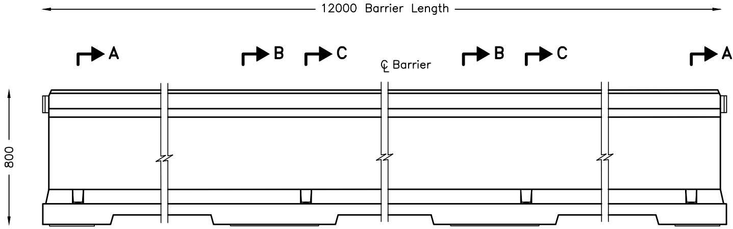
ELEVATION
